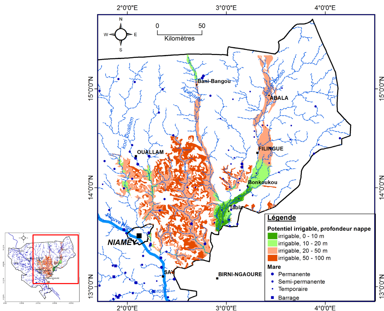
Fig. 3. Potentiel de terres irrigables suivant la profondeur de la nappe phréatique.
